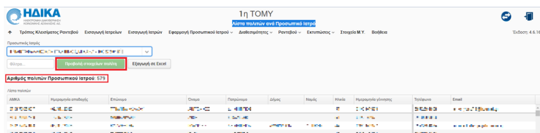
Εικόνα 9: Λίστα πολιτών
