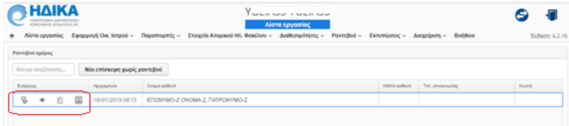
Εικόνα 2: Λίστα εργασίας
