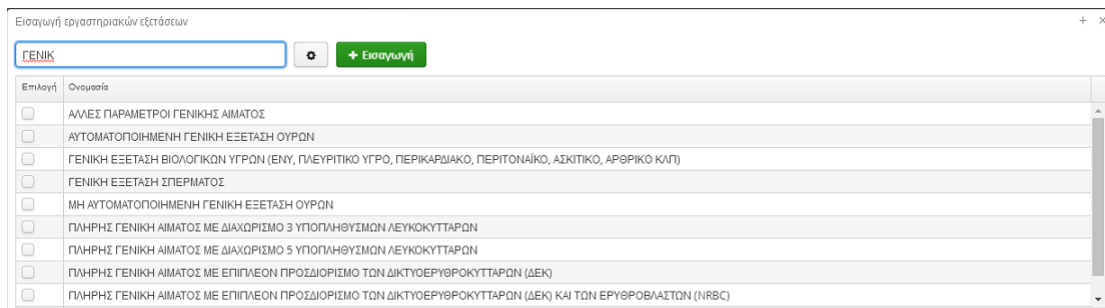
Εικόνα 36: Αναζήτηση-Εισαγωγή εξέτασης
